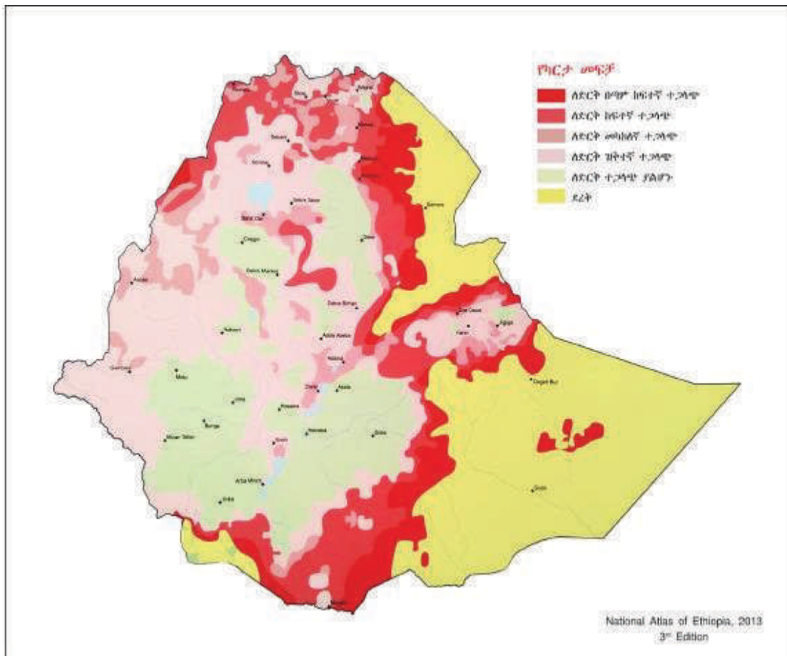
ስዕል 2 - በኢትዮጵያ የድርቅ ተጋላጭ ቦታዎች
